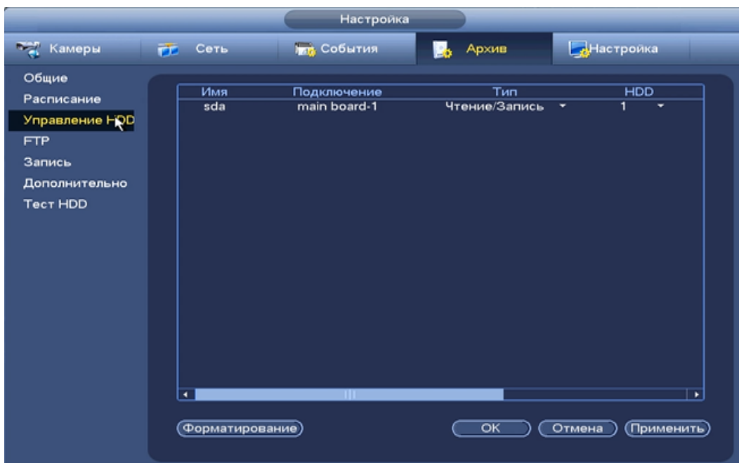
Рисунок 8.3.4.3.1 Интерфейс настройки
