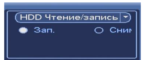
Рисунок 8.1.3.1 Тип поиска
