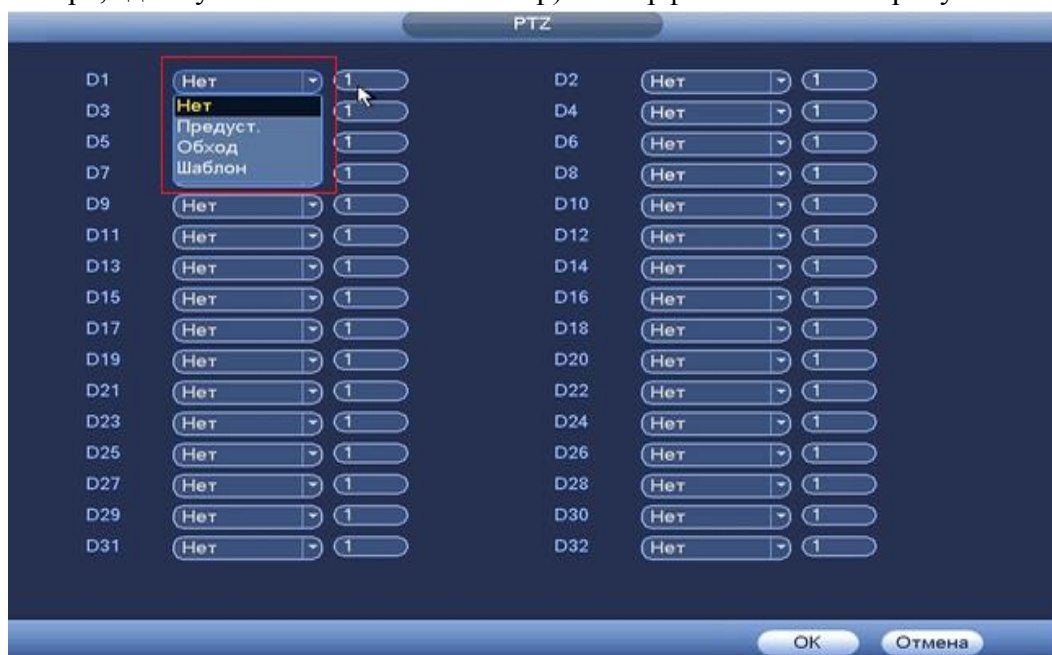
Рисунок 8.3.3.4.5 Установка предустановок.
