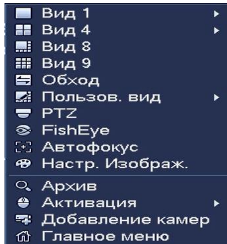
Рисунок 7.1 Контекстное меню.
