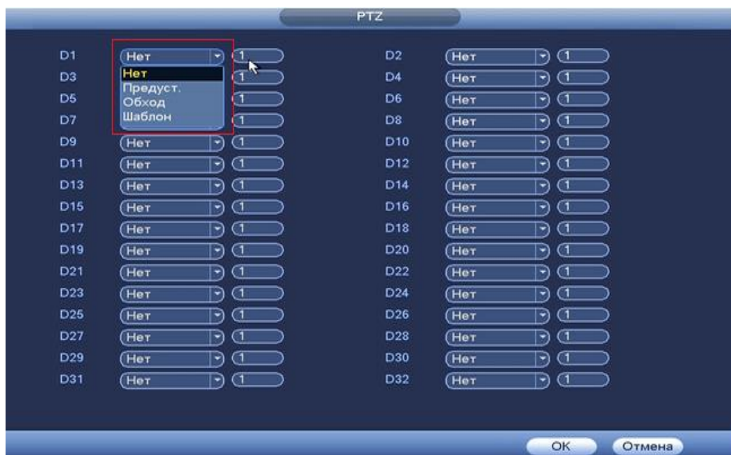
Рисунок 8.3.3.3.5 Установка предустановок.
