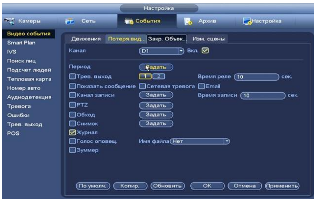
Рисунок 8.3.3.1.2.5 Установка настроек.
