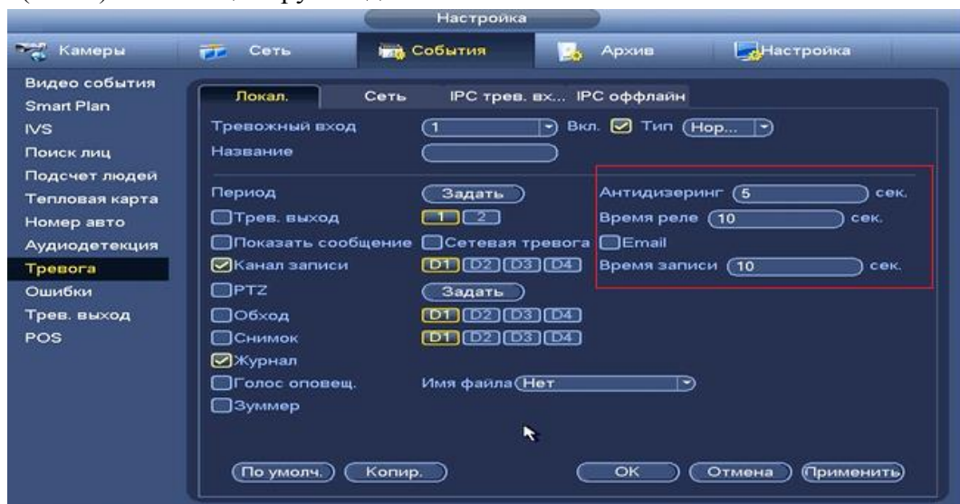
Рисунок 8.3.3.9.1.5 Установка настроек.
