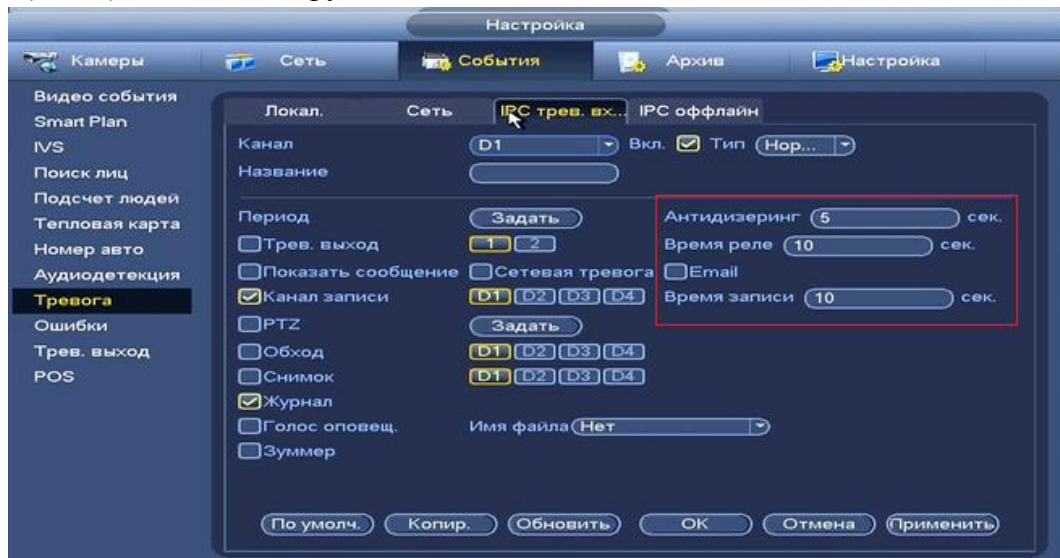
Рисунок 8.3.3.9.3.5 Установка настроек.
