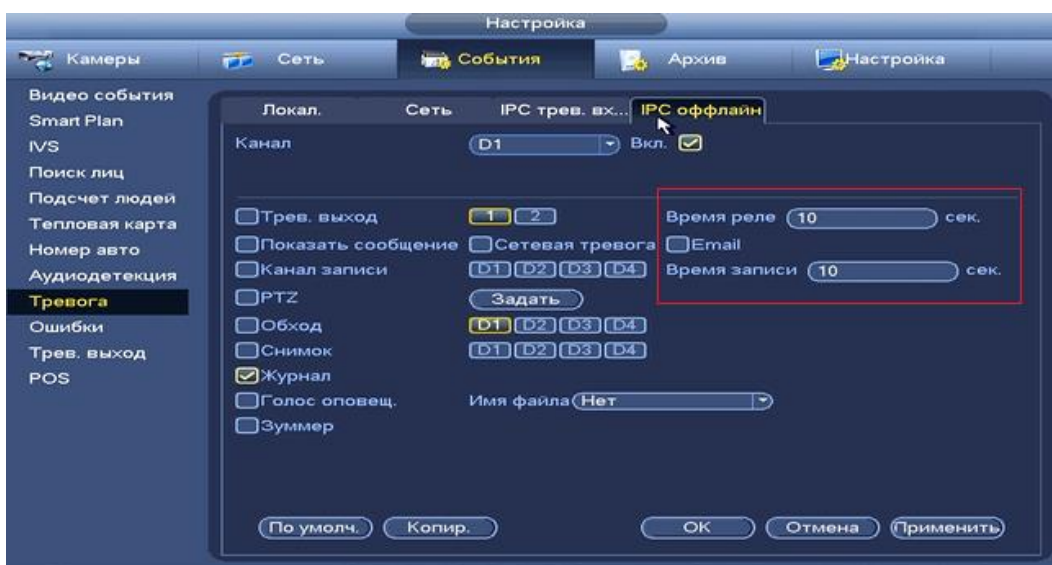
Рисунок 8.3.3.9.4.3 Установка настроек
