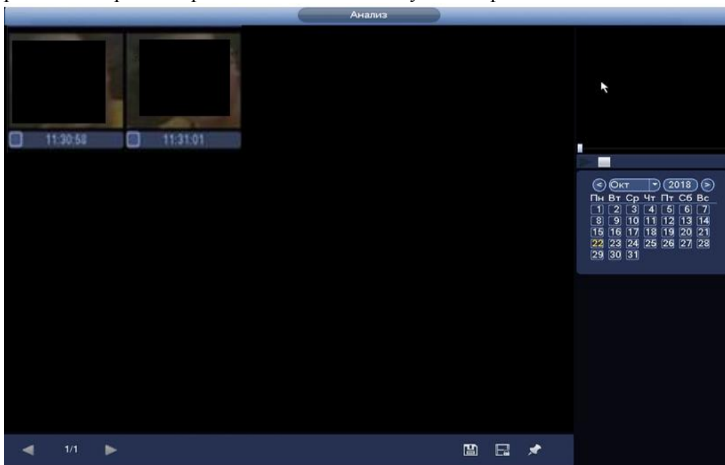
Рисунок 8.1.2.2.1 Распознавание лиц.
