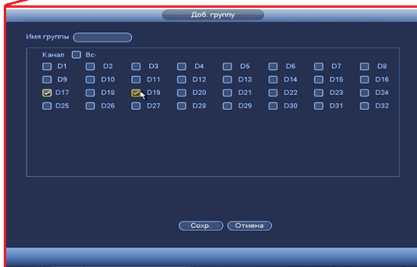
Рисунок 8.3.4.5.1.1 Добавление группы.
