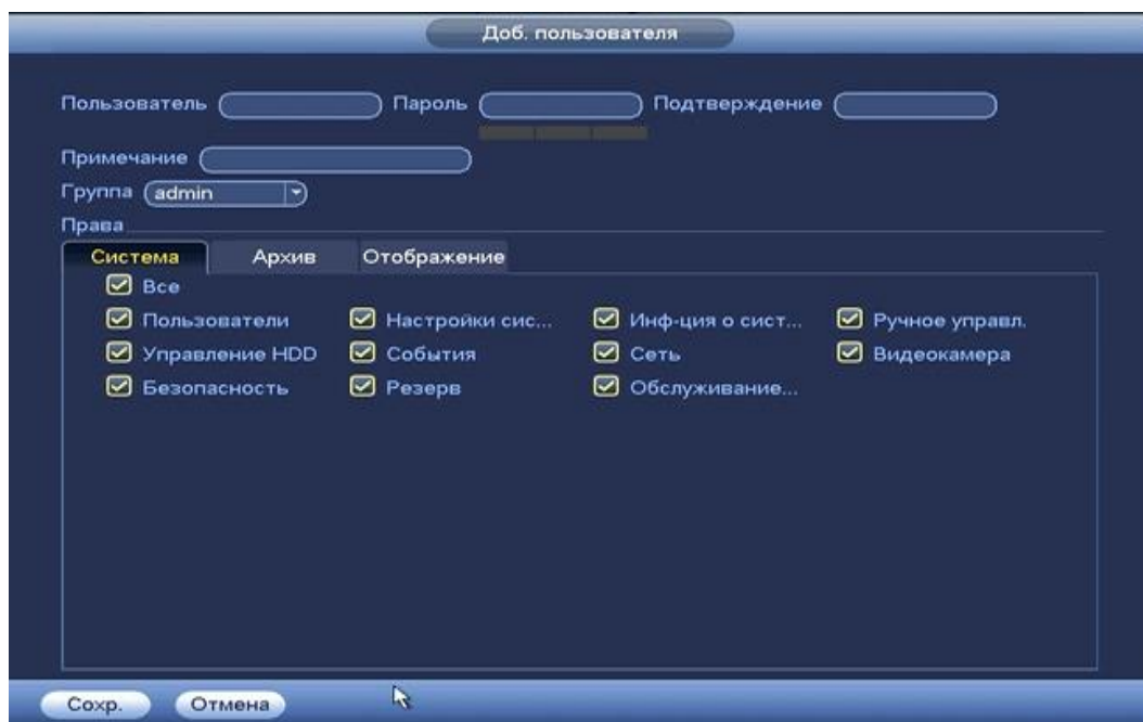
Рисунок 8.3.4.5.1.2 Назначение прав.
