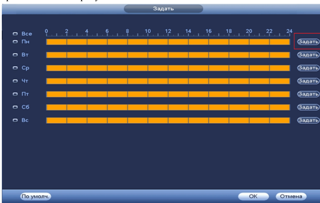
Рисунок 8.3.3.3.3 Настройка расписания.
