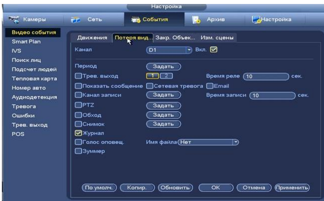
Рисунок 8.3.3.1.3.5 Установка настроек.
