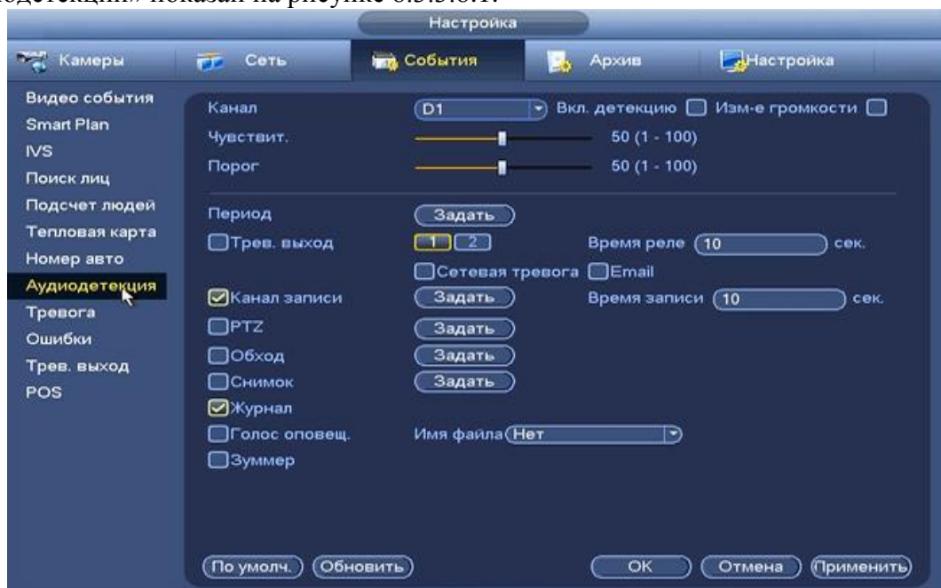
Рисунок 8.3.3.8.1 Настройка аудиодетекция.
