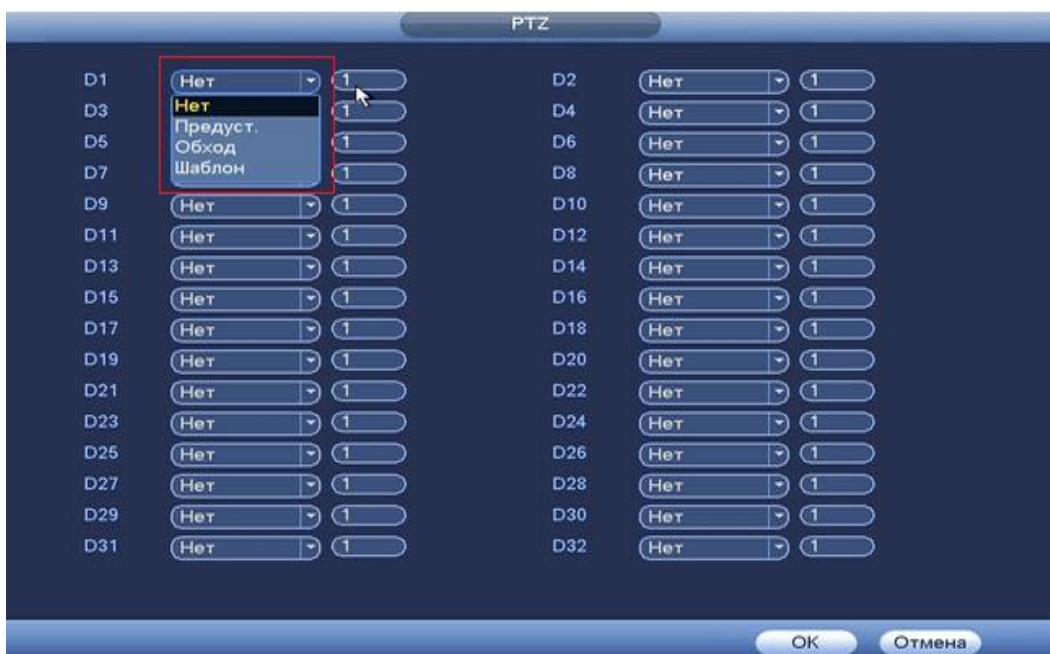
Рисунок 8.3.3.5.4 Установка предустановок.
