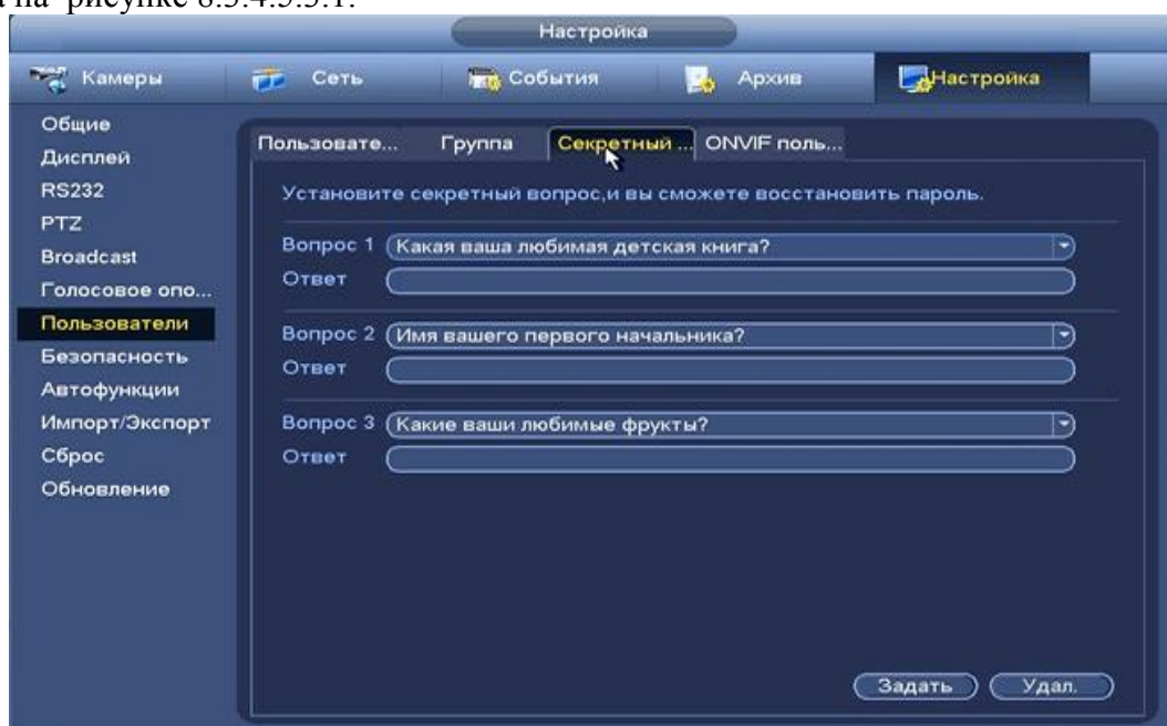
Рисунок 8.3.4.5.3.1 Интерфейс настройки
