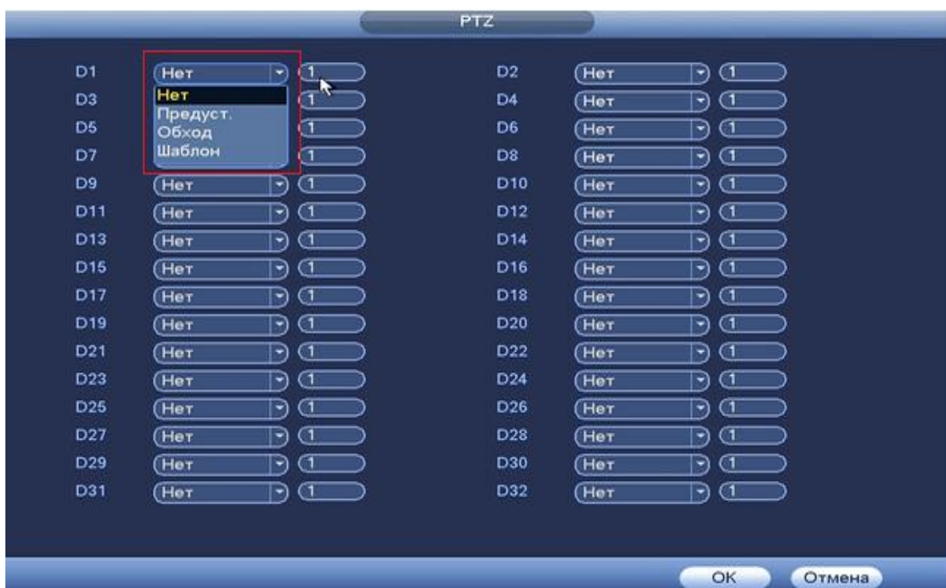
Рисунок 8.3.3.3.2.5 Установка предустановок.
