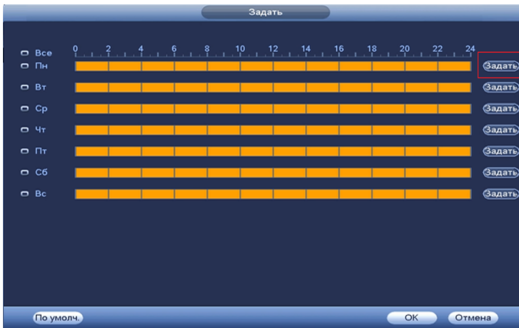
Рисунок 8.3.3.1.3.2 Настройка расписания.
