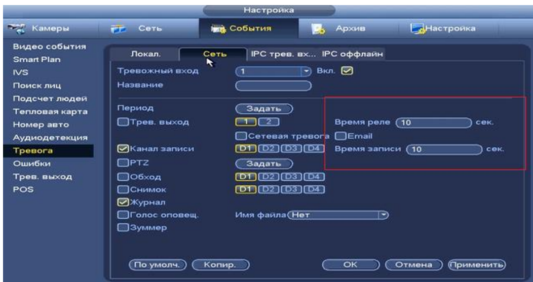
Рисунок 8.3.3.9.2.5 Установка настроек.
