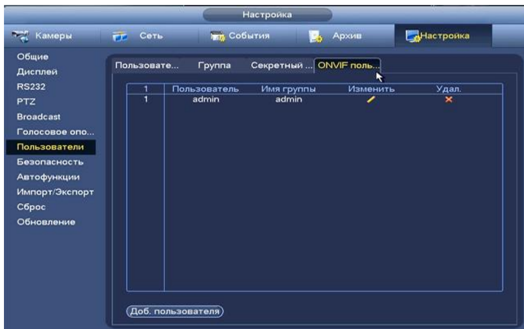
8.3.4.5.3.1 Настройка ONVIF.
