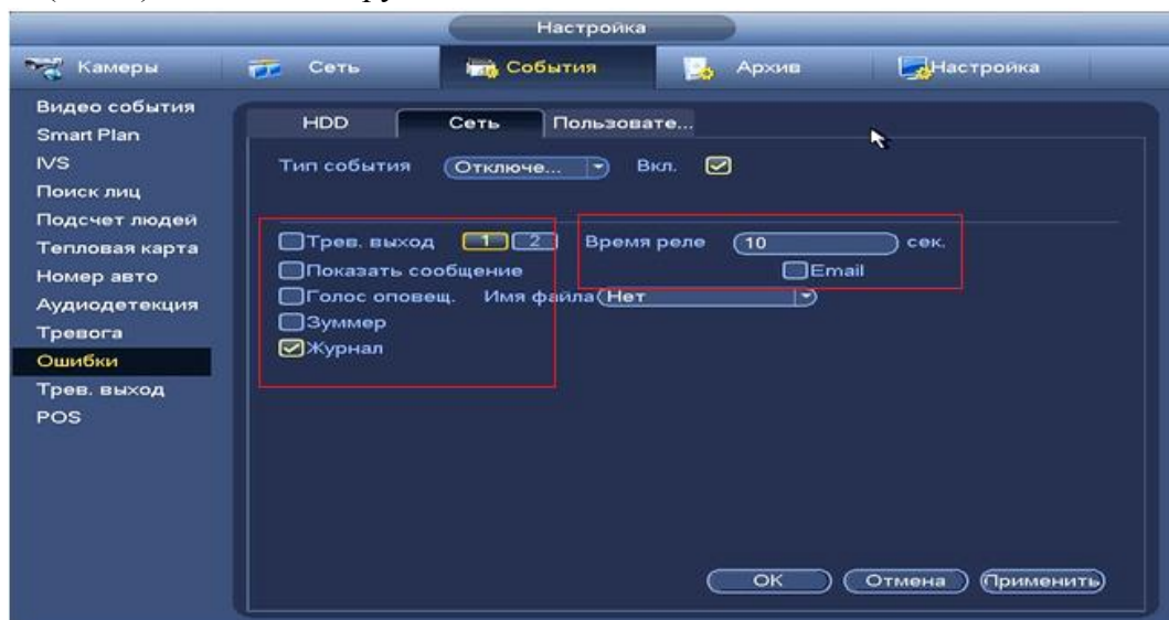
Рисунок 8.3.3.10.2.2 Установка настроек.
