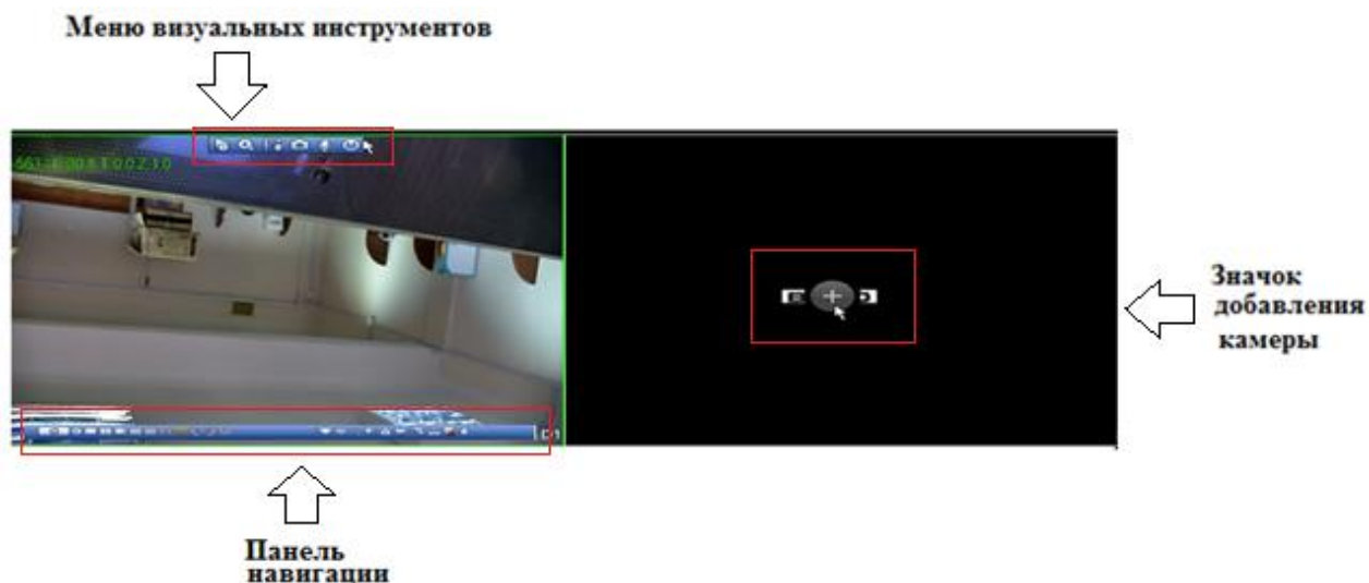
Рисунок 7.1.1.1 Добавление IP-камер.
