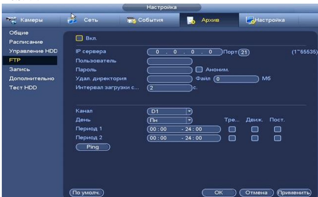
Рисунок 8.3.4.4.1 Настройка FTP
