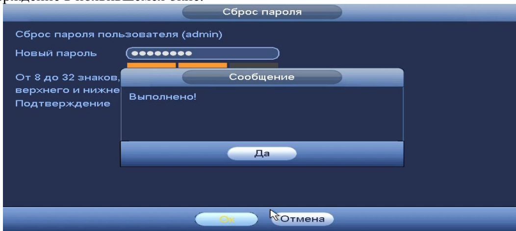
Рисунок 8.4.2.3 Ввод пароля.
