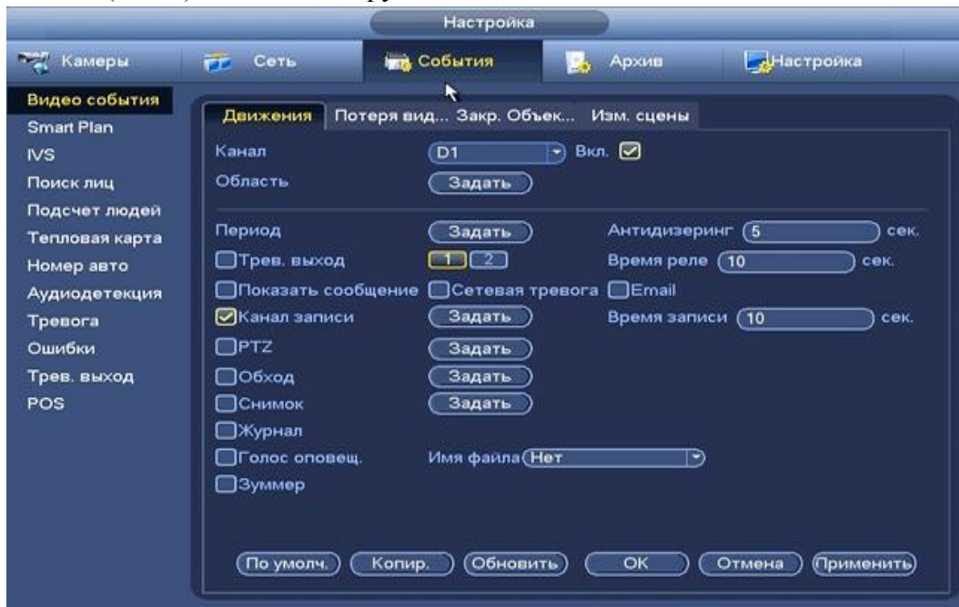
Рисунок 8.3.3.1.1.6 Установка настроек
